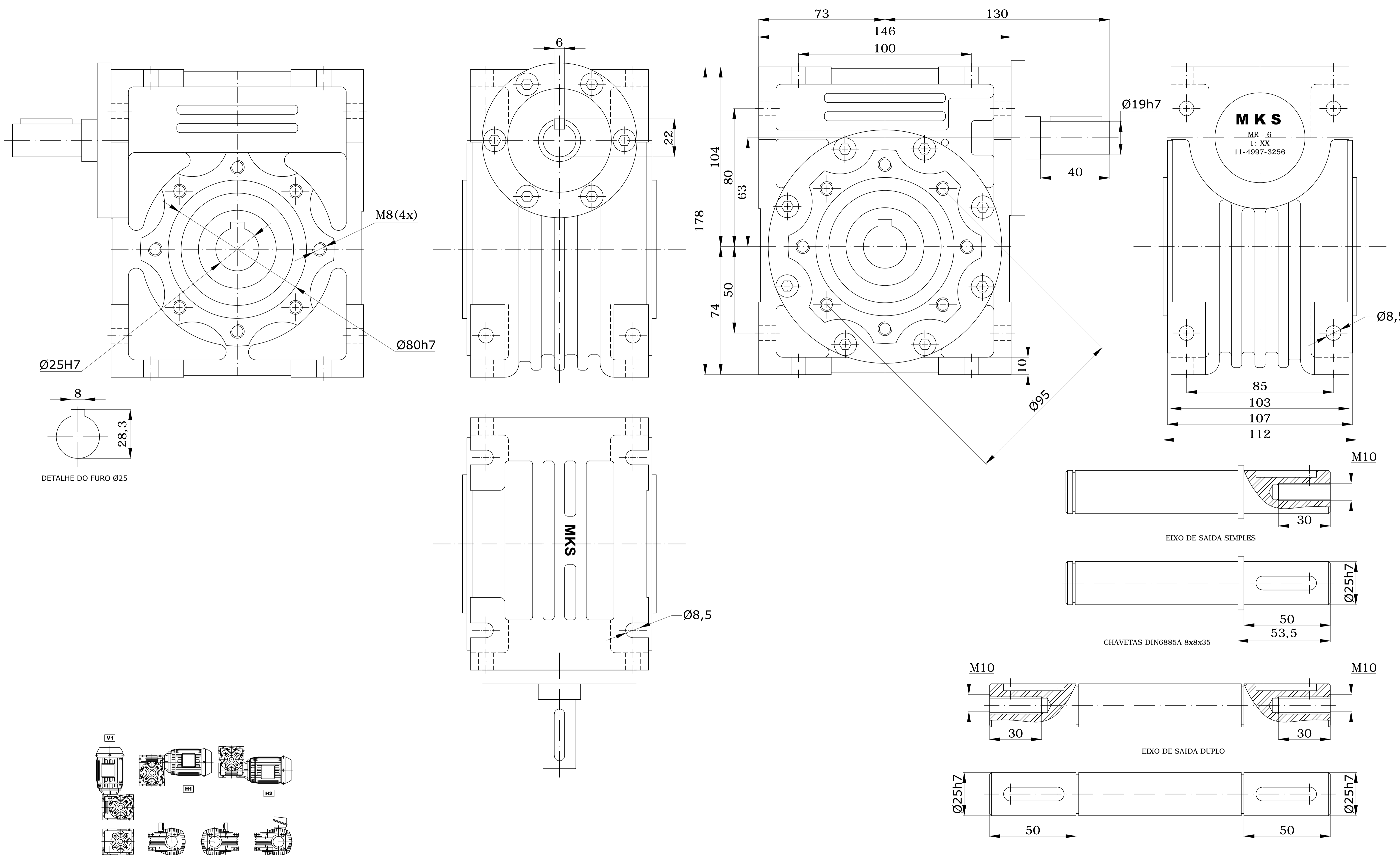
POSIÇÕES DE MONTAGEM SEM ESCALA
